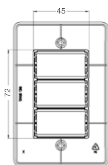
Placa 4x4 - 6 Posições
