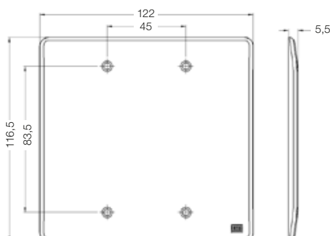
Placa 4x4 - Cega
