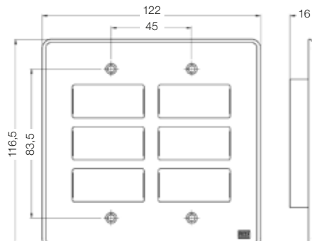
Placa 4x4 - 6 Posições
