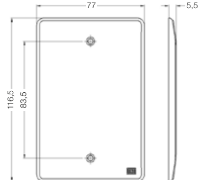
Placa 4x2 - Cega
