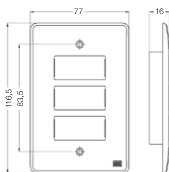
Placa 4x2 - 3 Posições
