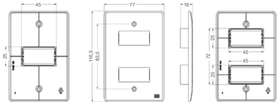
Placa 4x2 - 2 Posições
