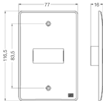
Placa 4x2 - 1 Posição
